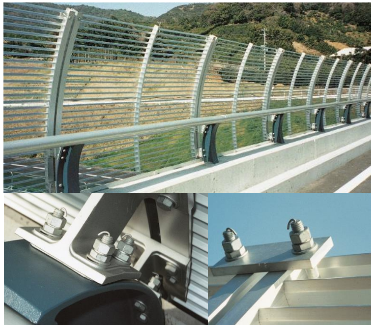
アルミ製投物防止柵（第二東名高速）
