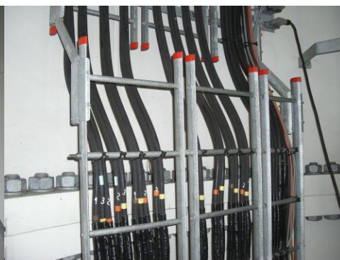
風力タワー内部配管
